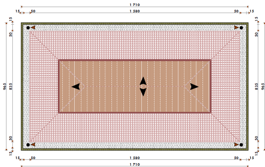
PLAN DE TOITURE - ROOF PLAN
