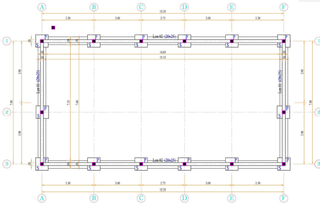
PLAN DE FONDATION - FOUNDATION PLAN
