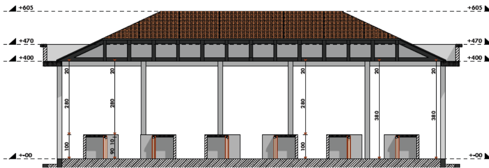
COUPE AA - SECTION AA
