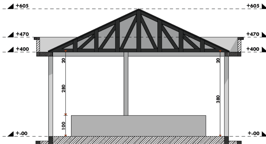
COUPE BB - SECTION BB
